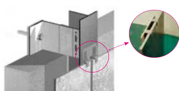
FACHADA COM GRAMPO À VISTA FACADES USING VISIBLE FASTENERS FAÇADE AGRAFÉE AVEC AGRAFE APPARENTE FACHADA CON GRAPA A LA VISTA
