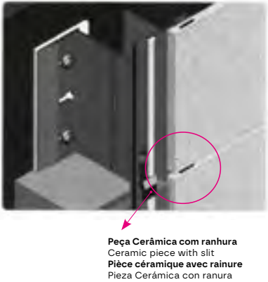
FACHADA COM GRAMPO OCULTO FACADES USING HIDDEN FASTENERS FAÇADE AGRAFÉE AVEC AGRAFE OCCULTE FACHADA CON GRAPA OCULTA
