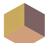
TRIO SUNSET BREEZE (a) (f) Cromática: Ocre + Malva + Coral 20x22x0,85 cm SOFT P22/peça_pieça [ 1m² = 32 peças_pieças ]
