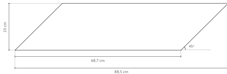
CHEVRON 20x90 cm [1m 2 = 7 peças_pieces]
