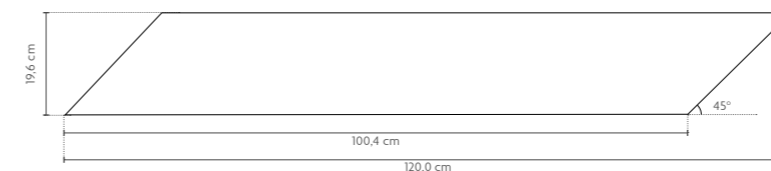
CHEVRON 19,5x120 cm [ 1m 2 = 5 peças_pieces ]
